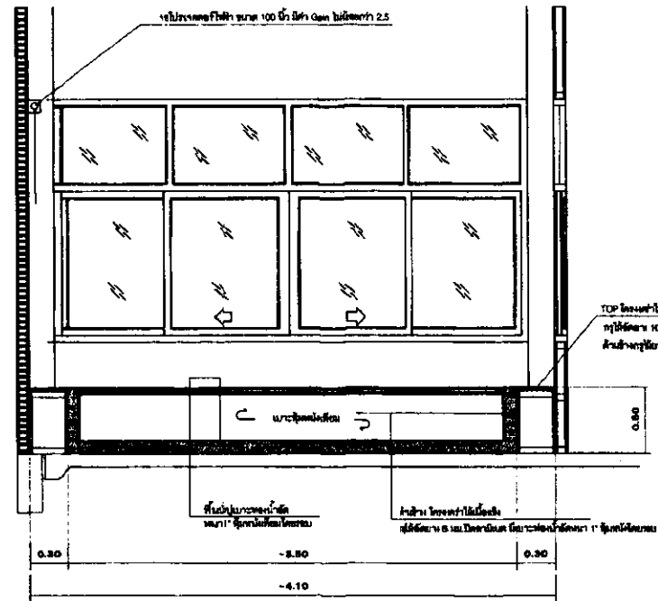
แบบขยายรูปตัดเฟอร์นิเจอร์ F-3 1:25
