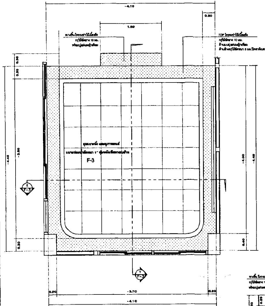
แบบขยายเฟอร์นิเจอร์ F-3 1:25
